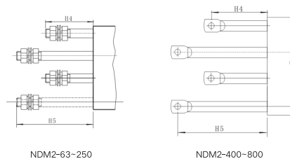
图 2 板后接线/ Fig 2 Rear connection
