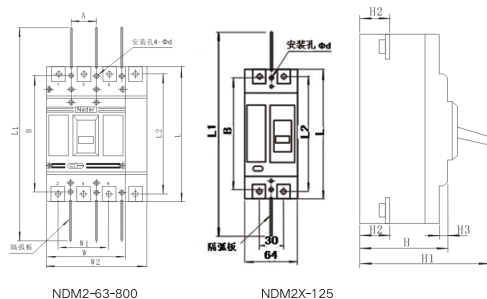
图 2 板后接线/ Fig 2 Rear connection
